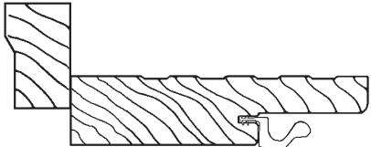
5 3 / 16 " Primed Jamb
