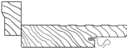
6 9 / 16 " Primed Jamb
